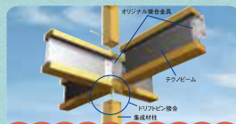
木+鉄のオリジナル複合梁テクノビーム
